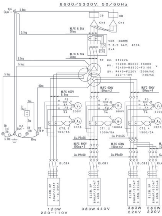
■ TTS-X510 結線
