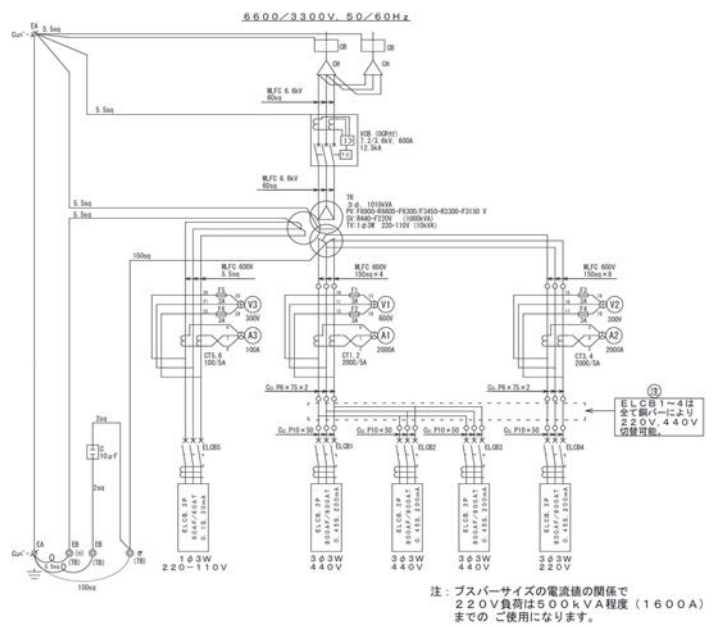
■ TTS-X1010 結線
