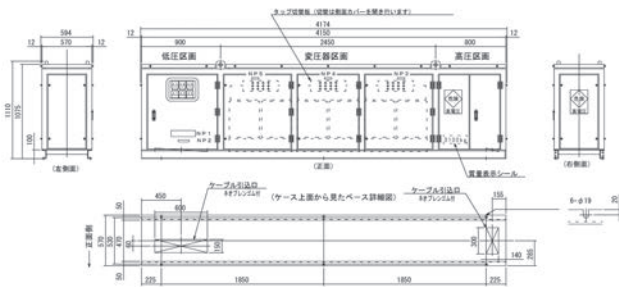
■ TTS-X510 外形図
