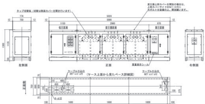
■ TTS-X1010 外形図
